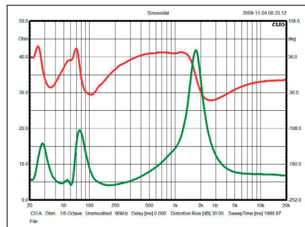
Typisk, snällt hög refleximpedans (grön). Som lägst 4,5 Ohm vid 60 och runt 180 Hz. Fäsväxlingarna (röd) kunde dock varit lite mjukare i basen och kringdelningen vid 2 kHz.
