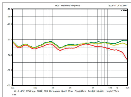
System Audio har aningen svajig, men tätt samlad frekvensgång mätt horisontellt vid 0° (grön) och 30° (gul). Diskantfallet börjar först vid 60° (röd), men snyggt och kontrollerat.
